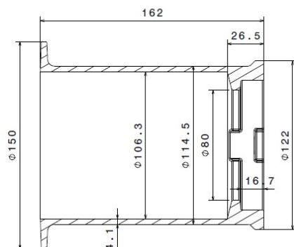
Section view B-B Scale: 2:3
